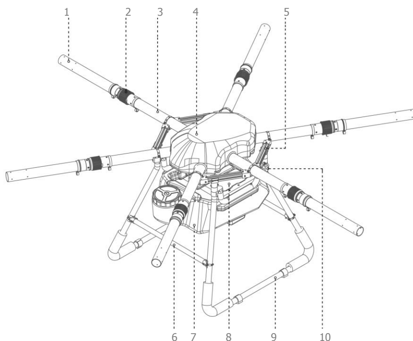
(上图)附图 3.机架模块结构 图 3
